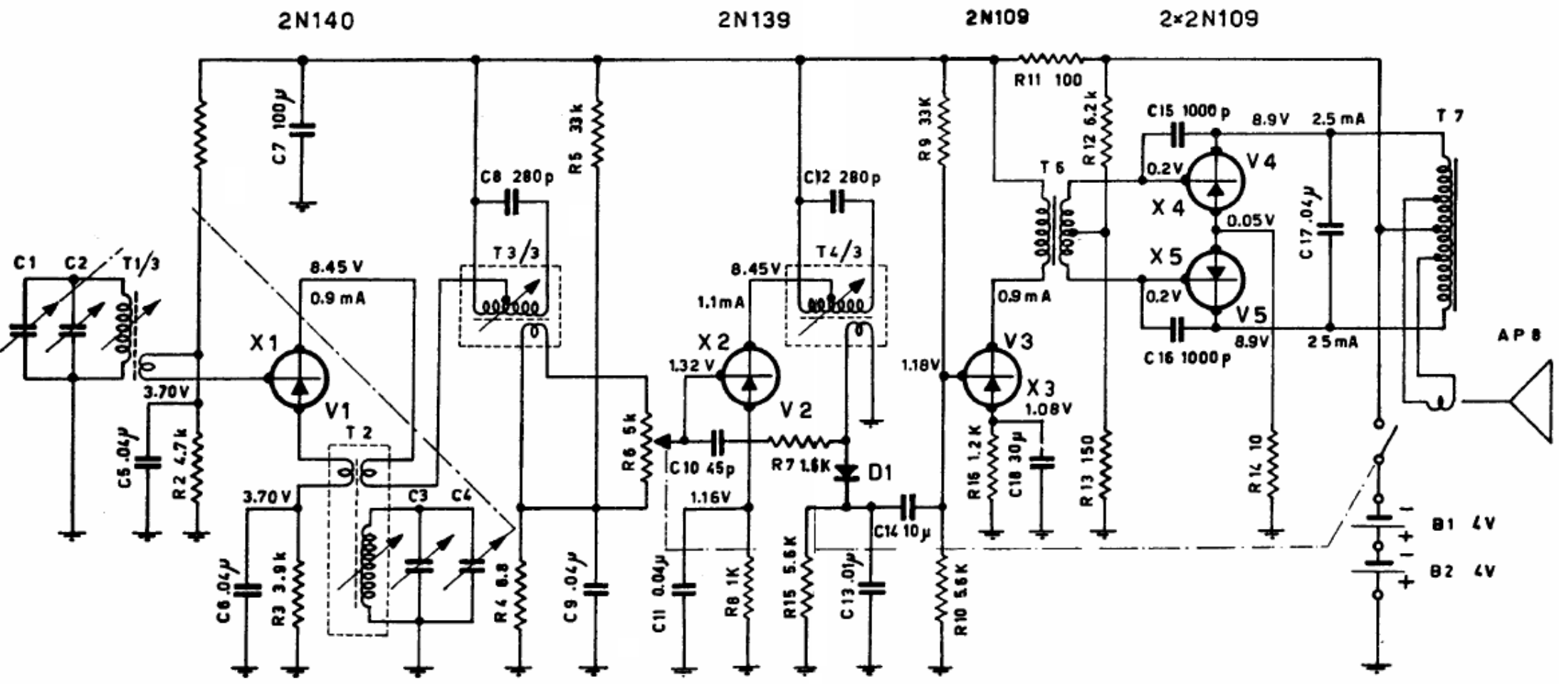
AUTOVOX - Mod. RT-53. Apparecchio portatile a 5 transistori e un diodo al germanio. Gamma di ricezione: onde medie da 530 a 1600 kc/s, Media frequenza a 455 kc/s. Consumo senza segnale: 10 mA. Alimentazione a 9 volt. Durata autonomia: 75 ore con batterie al biossido, 250 ore con batterie al mercurio. Altop. tipo AP8, da 86 mm.
